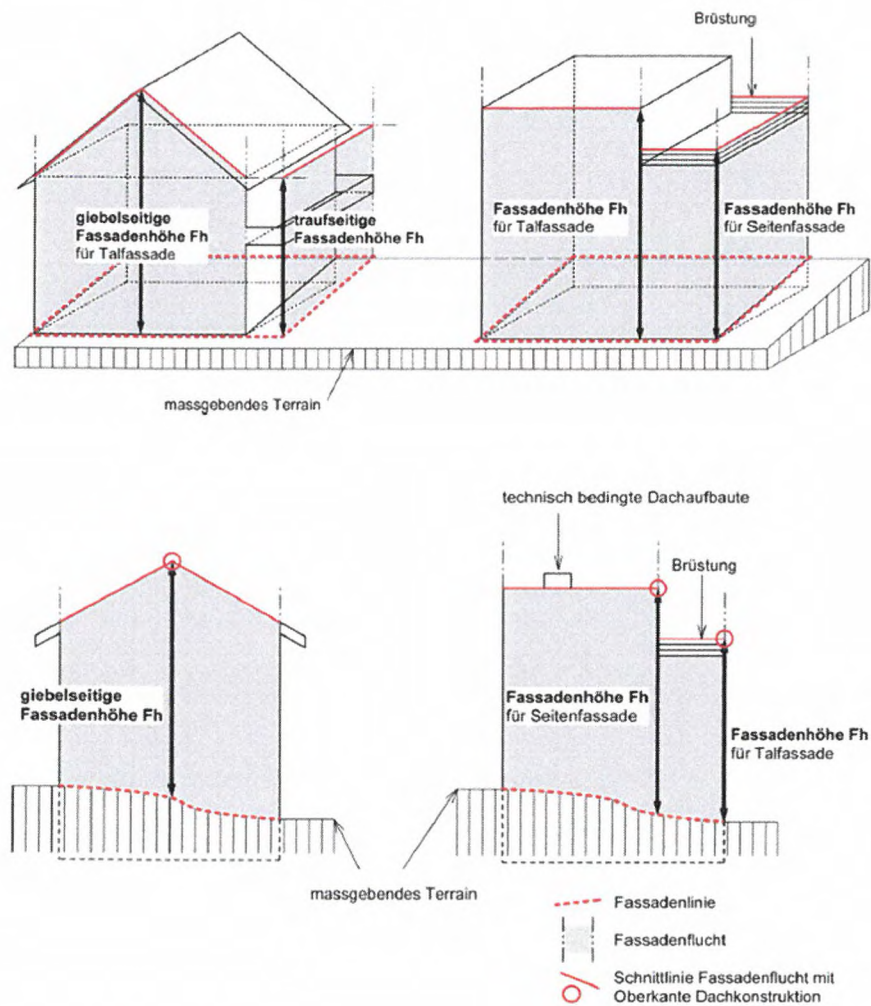
Figur 5.2 Fassadenhöhe
