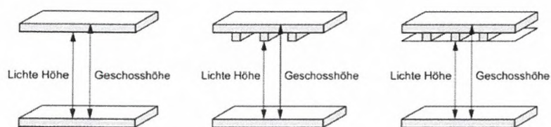
Figur 5.4 Lichte Höhe
