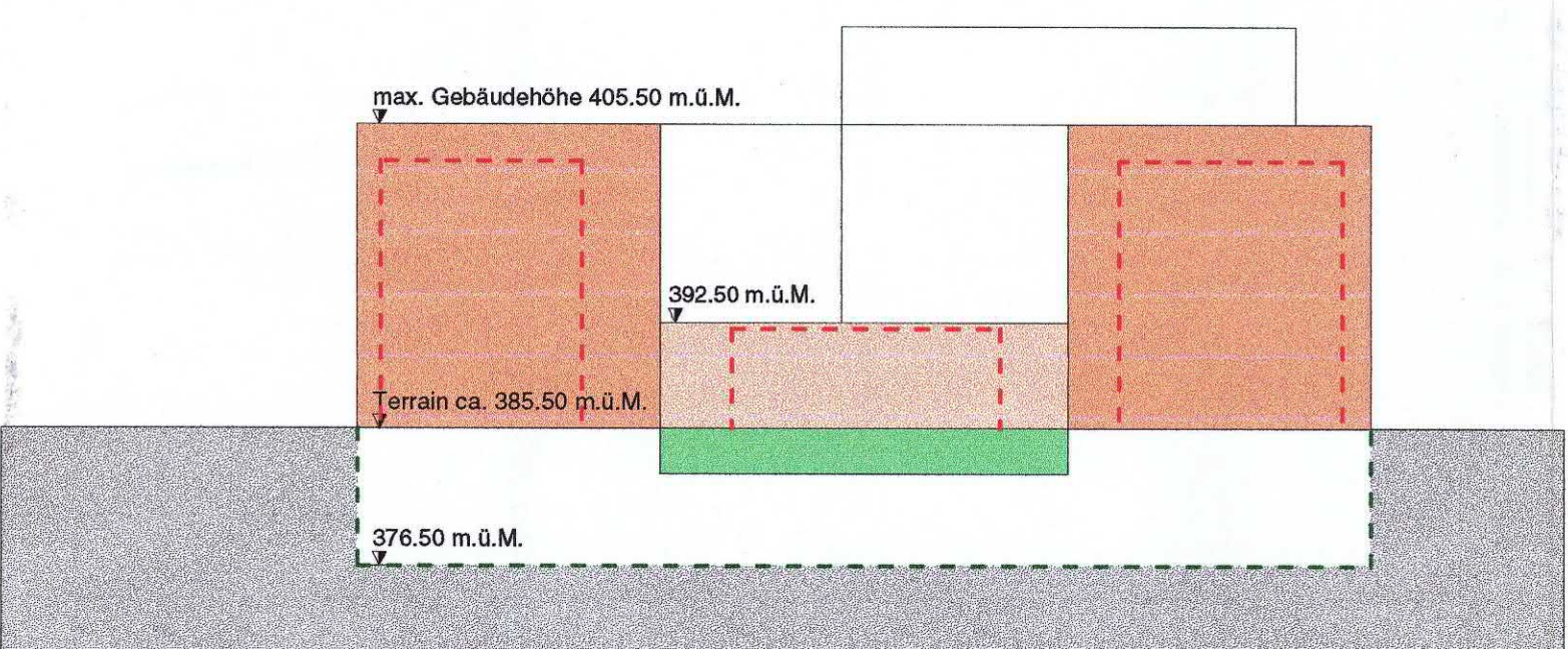
Querschnitt
