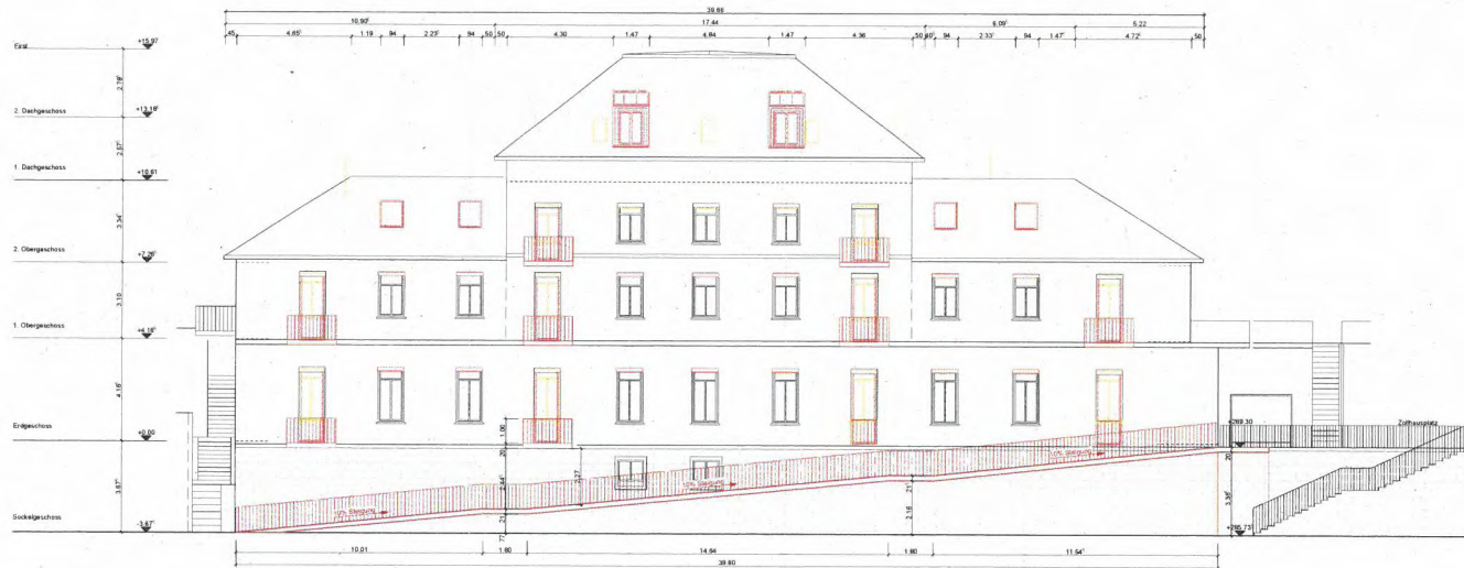
Westfassade 1:100
