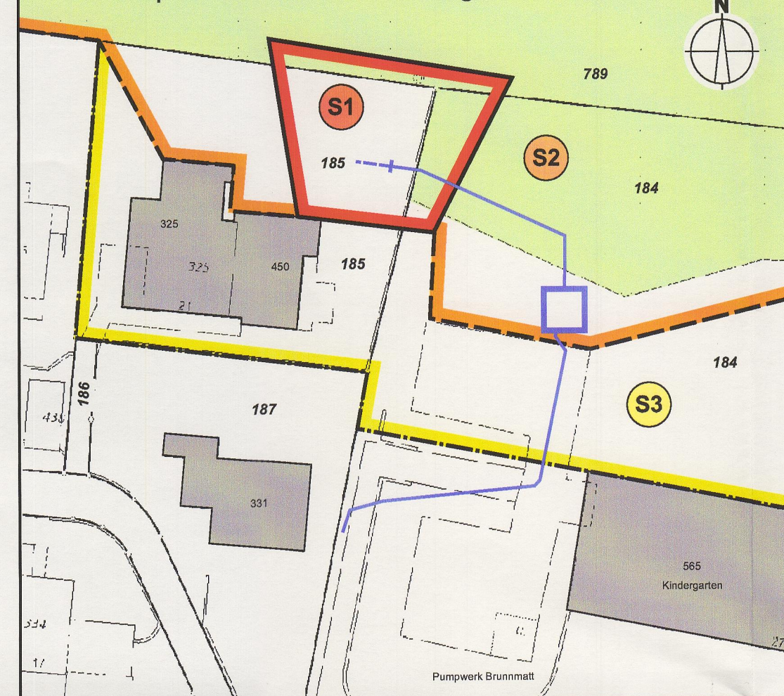
Detailplan Quellwasserfassung Brunnmatt 1:500
