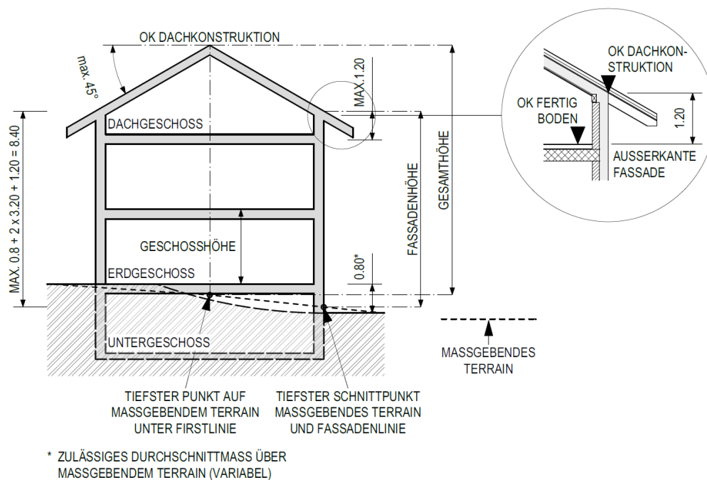
SCHRÄGDACH
