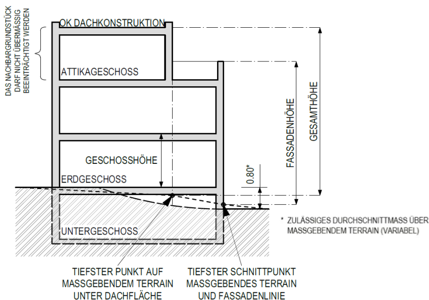
FLACHDACH MIT ATTIKAGESCHOSS
